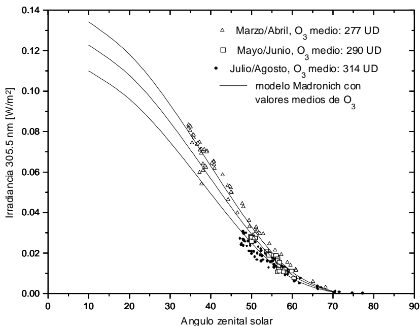
Figura 3. Irradiancia solar directa en 305.5 nm medida y modelizada en función del ángulo zenital, distinguiendo períodos bimestrales con sus correspondientes valores medios satelitales de ozono. Nota: las curvas se extendieron hasta el ángulo zenital mínimo para Rosario, de modo de dar una representación en otros períodos del año con valores de ozono similares a los indicados.
