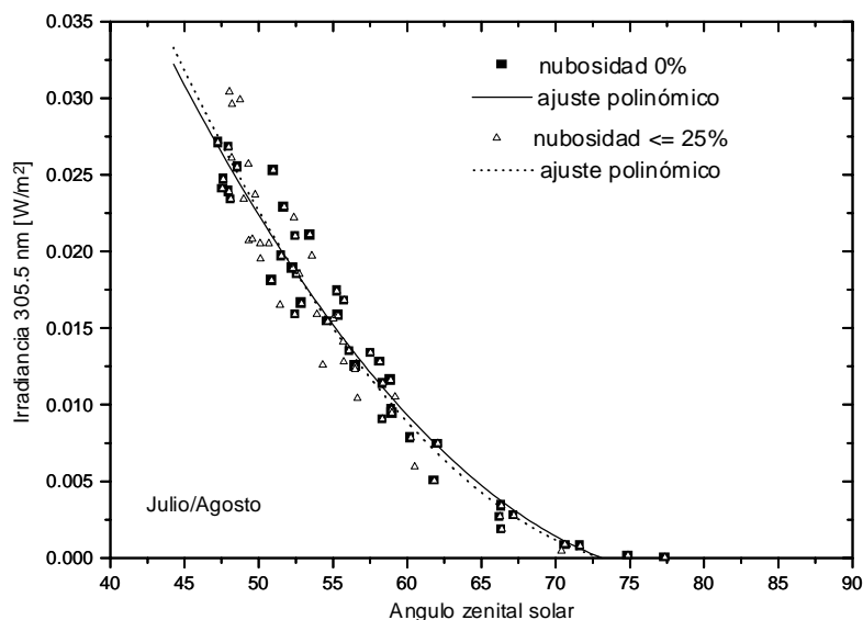
Figura 2. Irradiancia absoluta directa medida en 305.5 nm en función del ángulo zenital, distinguiendo los casos de nubosidad nula y nubosidad parcial, junto con los polinomios de ajuste correspondientes. Datos de julio-agosto 1998.
