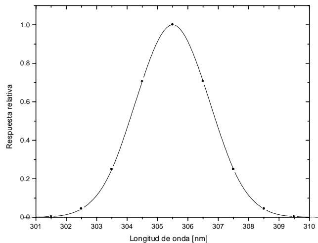
Figura 1. Función respuesta espectral utilizada en los cálculos teóricos, en correspondencia con las características del filtro espectral del instrumento.
