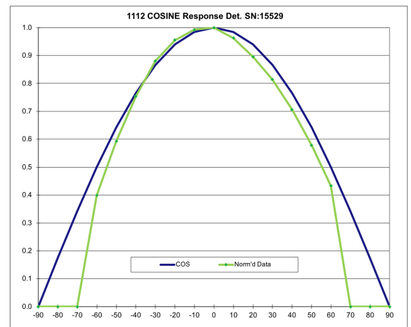
Fig. 4. Longitudinal Cosine Response
